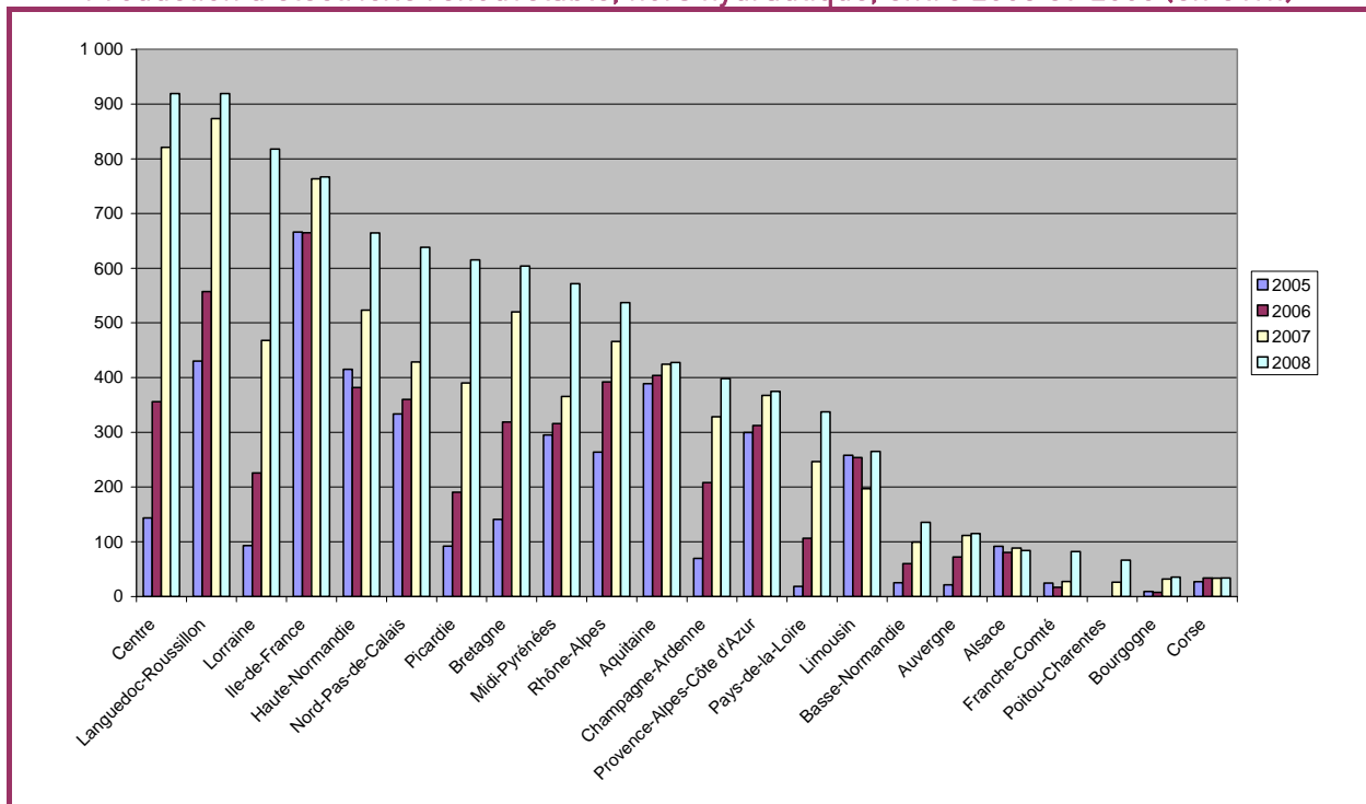
Production d'électricité renouvelable, hors hydraulique, entre 2005 et 2008 (en GWh)
